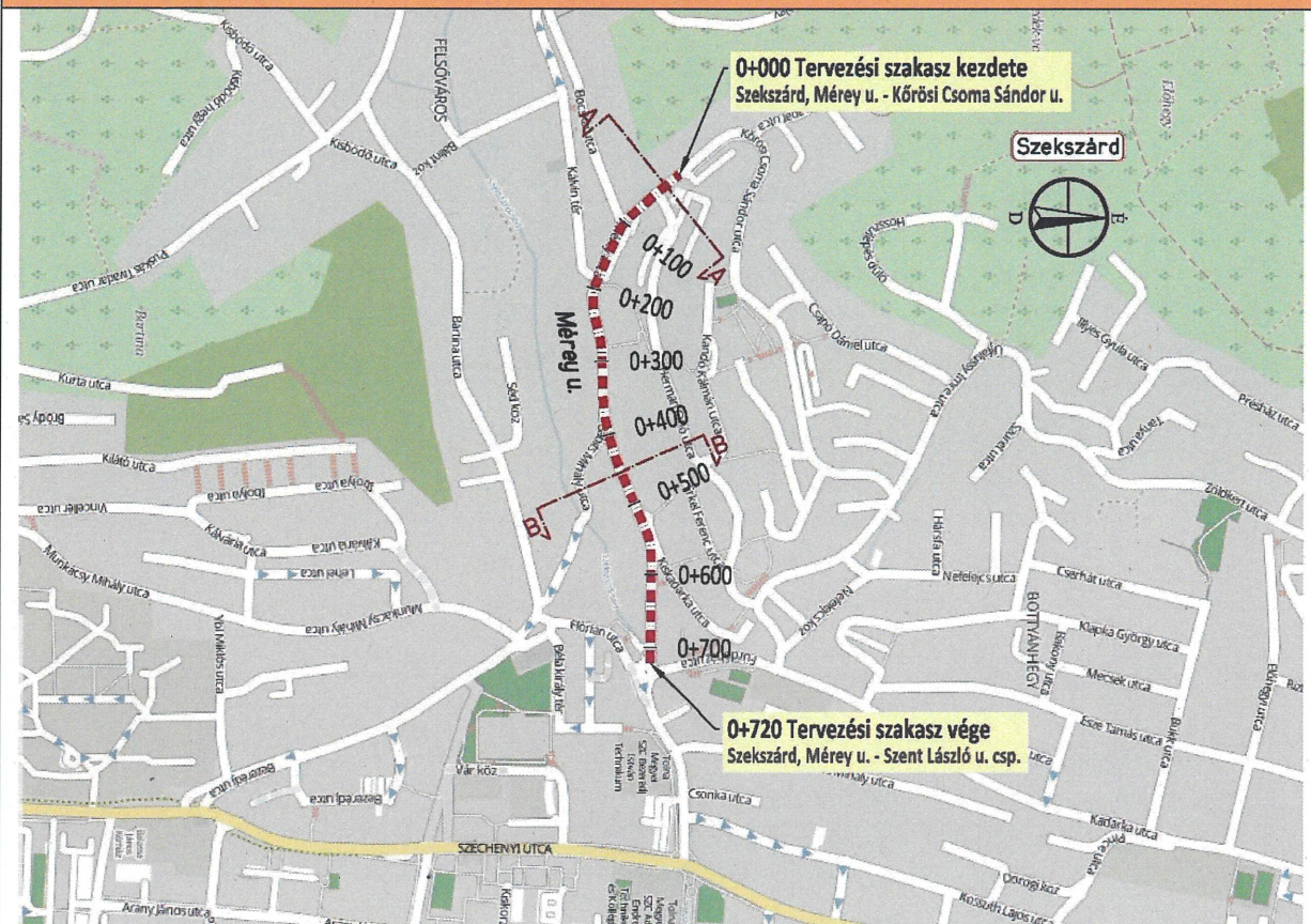
131. ábra: Helyszínrajzi elrendezés - Mérey utca (Körösi Csoma Sándor utca és a Szent László utcai körforgalom között)
