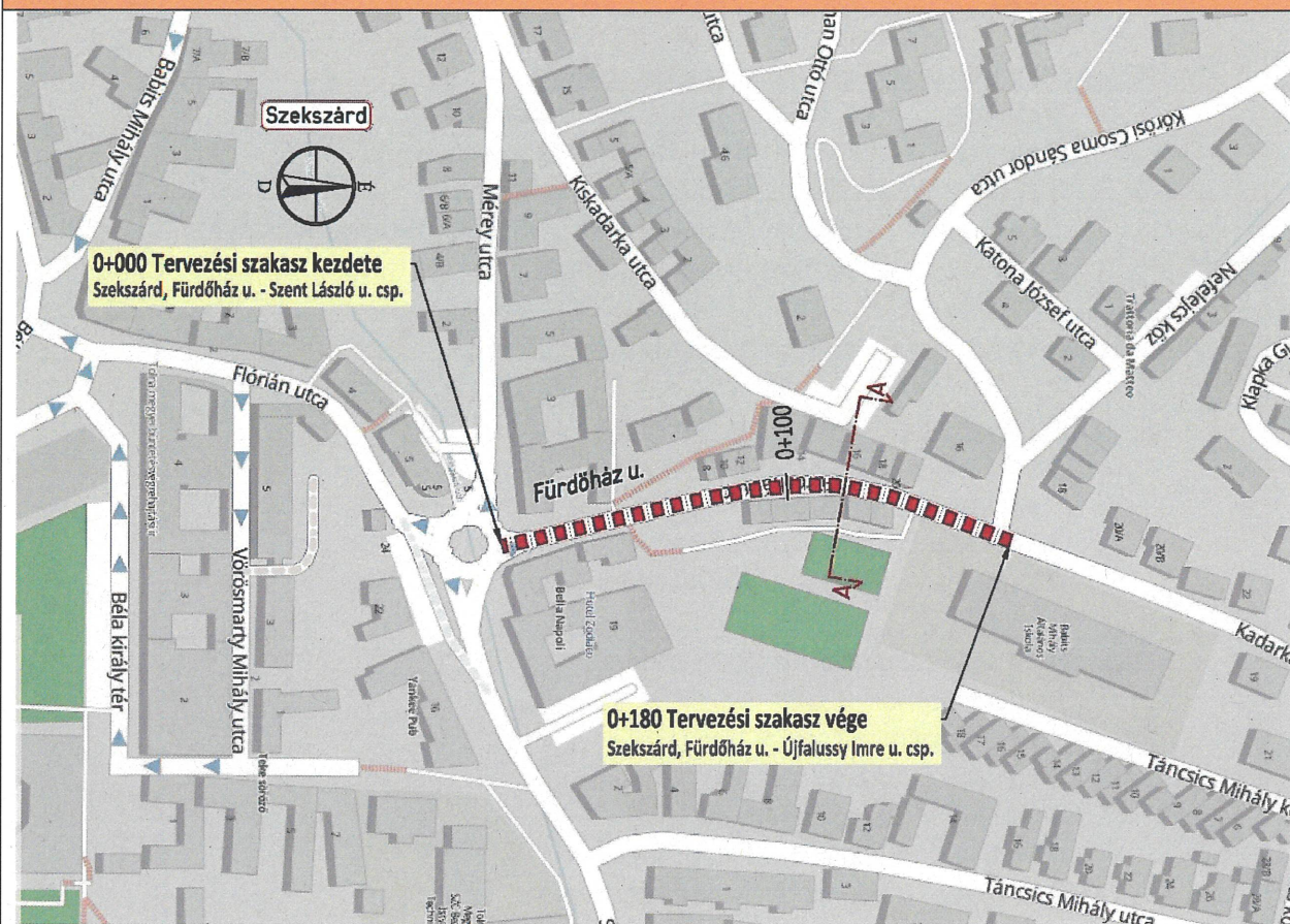
135. ábra: Helyszínrajzi elrendezés - Fürdőház utca (Szent László utcai körforgalom és az Újfalussy Imre utca között)
