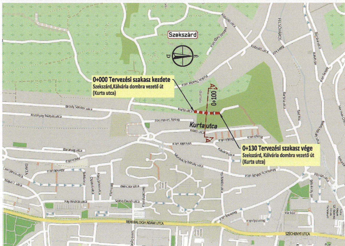
64. ábra: Helyszínrajzi elrendezés - Kálvária dombra felvezető út (Kurtajutca a köbburkolattal ellátott szakasza)
