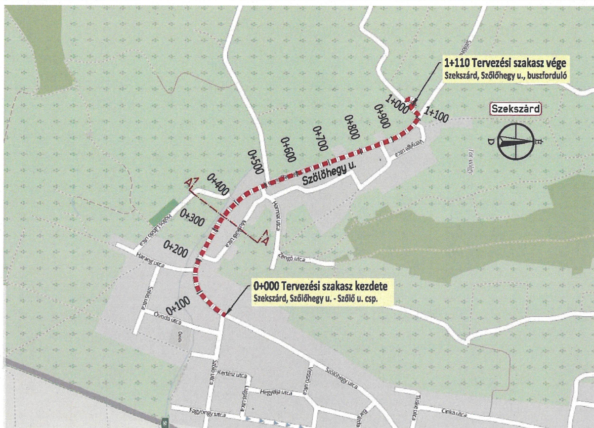
88. ábra: Helyszínrajzi elrendezés - Szőlőhegy utca (Szőlő utca és buszforduló között)
