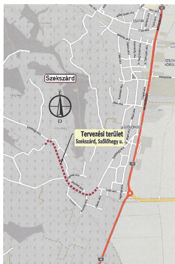
86. ábra: Átnézeti helyszínrajz - Szőlőhegy utca (Szőlő utca és buszforduló között)
