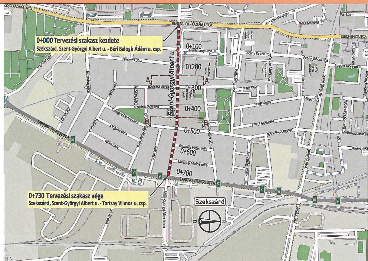
227. ábra: Helyszínrajzi elrendezés - Szent Györgyi Albert utca (Béri Balogh Ádám utca és a Tartsay Vilmos utca között)
